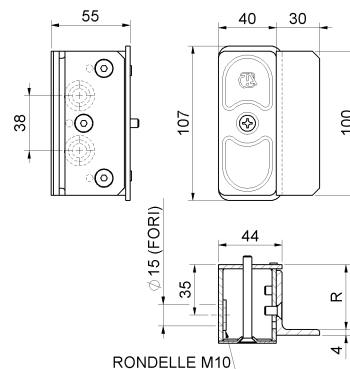
RONDELLE M10
